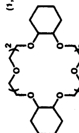
K 4 N 2 21C7-1 (±) K 4 N 2 21C7-2 (meso)
