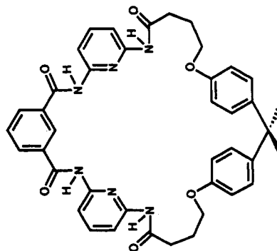
(1,3-B)(1,4-B) 2 Py 2 N 3 34C8-1
