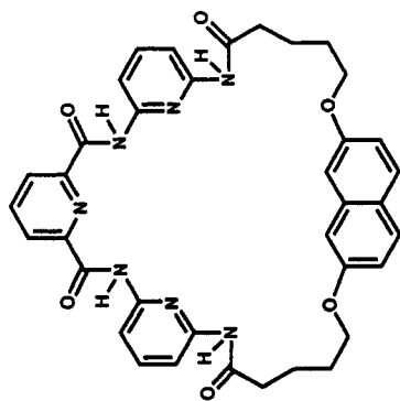
NapPy 2 N 3 32C8-1
