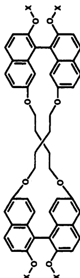
Nap 2 30C4-1 X = CH 2 CH 2 N(C 2 H 5 ) 2 + Cl - (RR)
