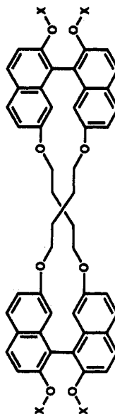
Nap-28C4-1 X = CH 2 CH 2 N(C 2 H 5 ) 2 + Cl - (HR)
